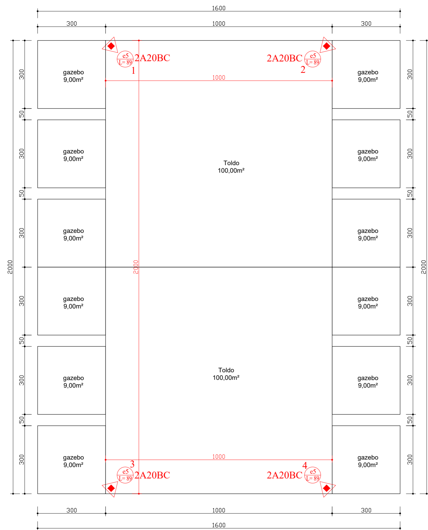
PLANTA BAIXA - ESTRUTURA MÓVEL ESC.: 1/100 - Á.: 308,00m²
